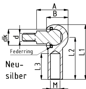
Winkelgelenk WG 5+6
