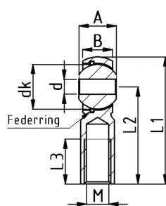
Gelenkkopf GKBF..
