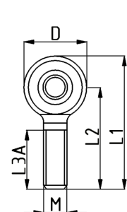
GKR..A mit Außengewinde
