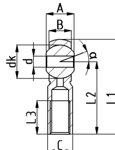
Gelenkkopf GKR ..
